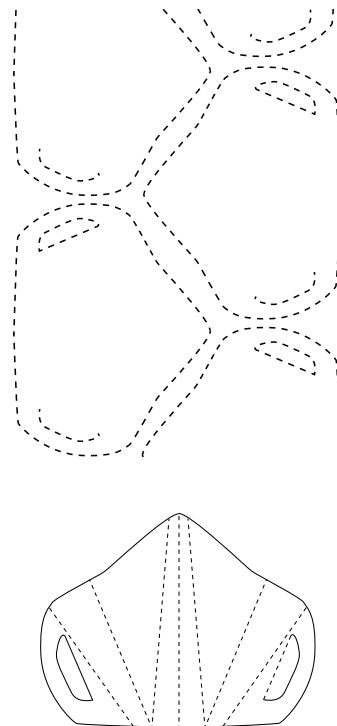
I den andra versionen stansas formen ut och går att passa ihop så att den ej borde ge mycket spillmaterial, sedan bigas den och viks innan den förpackas.
