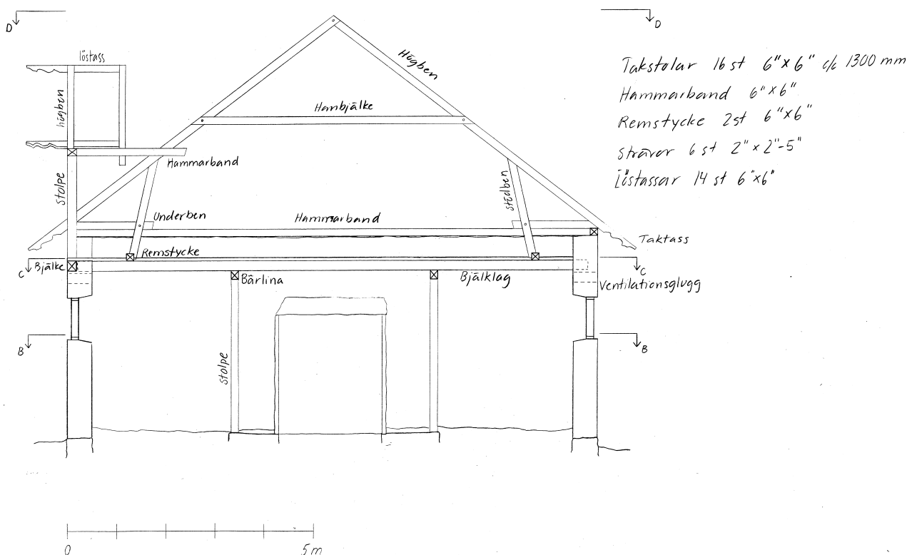
fig. 6 Uppmättningsritning med anteckningar om dimensioner och byggnadsdelar av Ann-Sofie Svensson.
