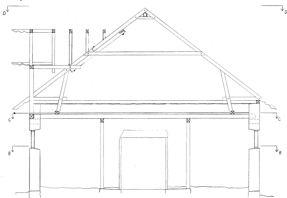
Bilaga V. Rekonstruktionsförslag på takkupa i snitt
