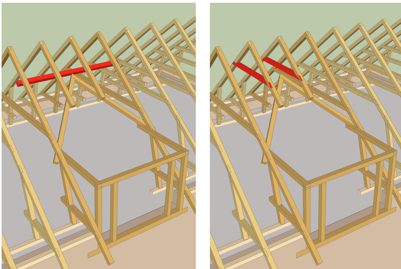
fig. 33 & 34, alternativa lösningar för att förstärka de mittersta takstolarna innan man sågar av dessa. Till vänster en rak avvaxling bultad fast på undersidan högbenen på de fyra takstolarna. Till höger hanbjälkar som styrar upp de två avsågade takstolarna. Spår av lösningar som liknar dessa har jag inte kunnat finna i resterna av konstruktionen, men det kan tyckas rimligt att vidta en åtgärd av detta slaget.
