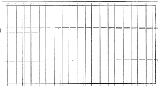
fig. 7 Överst takplan med takstolar, strävor, murrem och remstycken. Här saknas mötet mellan lastkupan och det övriga taklaget. Under visas ett plan men bjälkar och bärlinor. Uppmätningssritning av Ann-Sofie Svensson.
