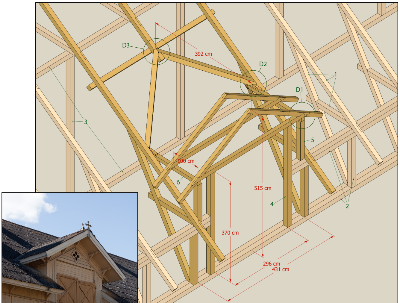
fig. 20 Uppmätning av lastkupan ovanför kostallet på Ryholm, Renritad i Google SketchUp.
