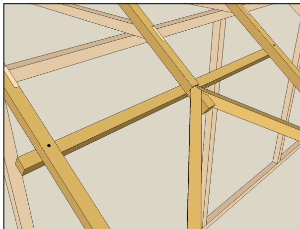
fig. 24 Detalj D3 enligt ritningen fig. 20. De båda kälsparrarna möter varandra på en avsågad takstol, som i sin tur får stöd av en avväxling.
