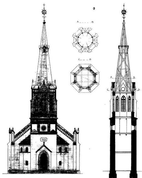
Ritning till ombyggnad av torn 1907. Tornet sträcker sig i fem våningar; nerifrån vapenhus, ett rum utanför läktare, tornvindsrum, klockrum samt rum i tornspiran. Bild Archidea AB.
