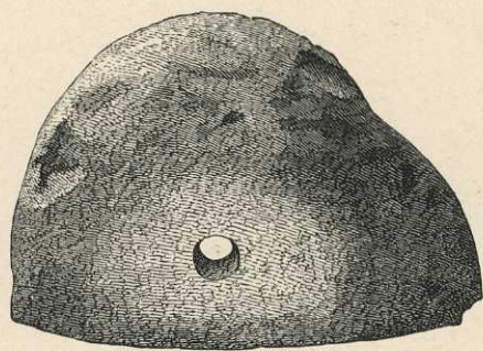
396 a. \frac{1}{3} 396 b. \frac{1}{3} 395. Avl-Sten. — Pierre servant de tuyère pour soufflet de forge.
