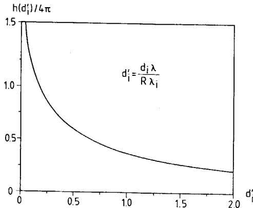
Figur 4.10.5. Värmeförlustfaktor för halvsfäriskt värmelager enligt figur 4.10.1.
