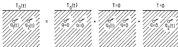
Figur 3.2. Superposition där ostörd marktemperatur och rena effektuttag för två yttjordvärmslangar separeras.
