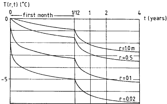
Figur 5.3.5. Temperaturutveckling på olika avstånd från röret för stegpulsens. Data enligt 5.3.2.3.
