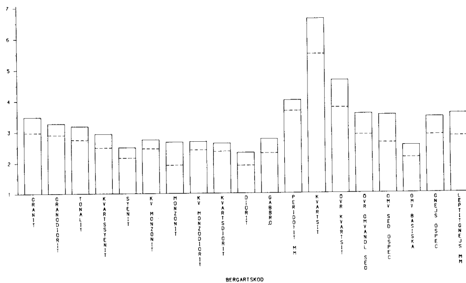
Figur 3.5. Värmeledning för kristallina bergarter
