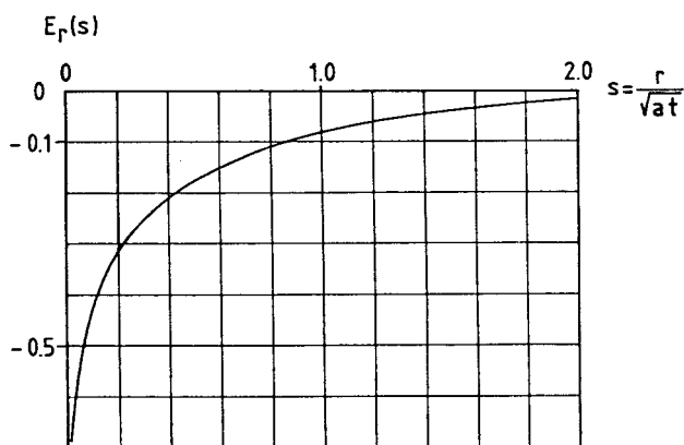
Figur 5.3.6. Temperaturprofilfunktion E_r(s) för stegpulsen.
