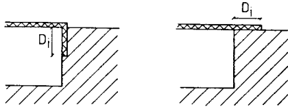
Figur 4.7.7. Vertikal kontra horisontell isolering vid kanten.
