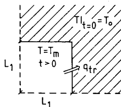
Figur 5.1.10. Transient process i ett plant tvärsnitt utanför ett hörn.
