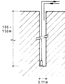
Figur 1.6. Bergvärmebrunn.
