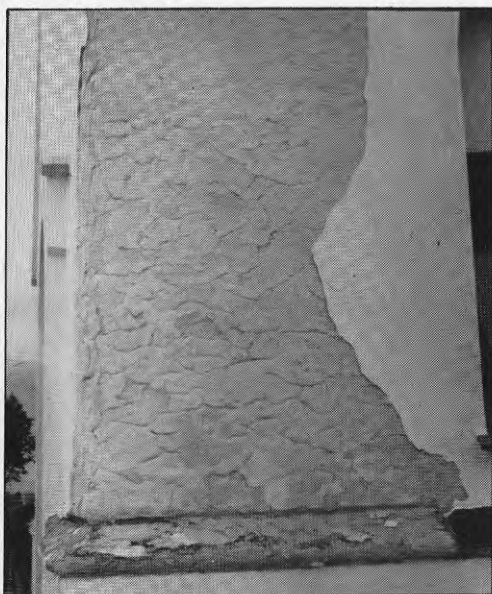
FIG. 5:18. Skadeutseende efter andra renoveringen, närbild.
