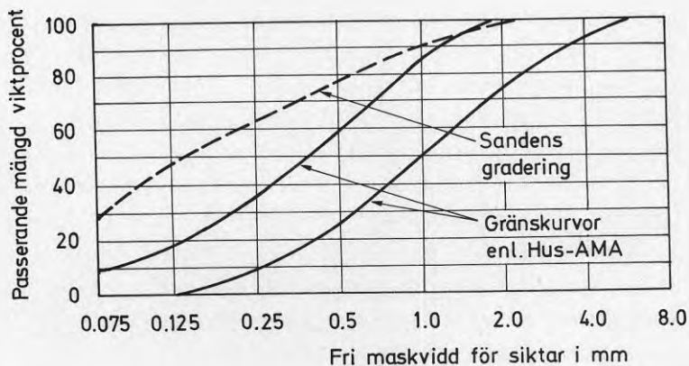
FIG. 5:1. Ballastgradering hos "putsanden".
