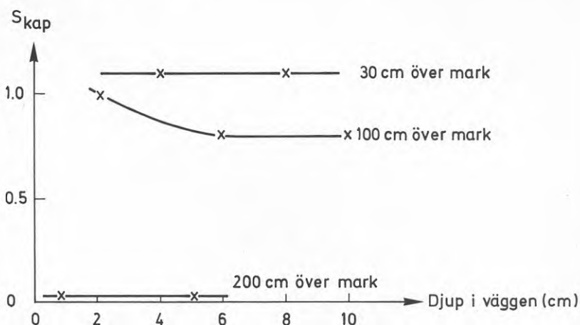
FIG. 5:6. Kapillära vattenmättnadsgrader i väggen.
