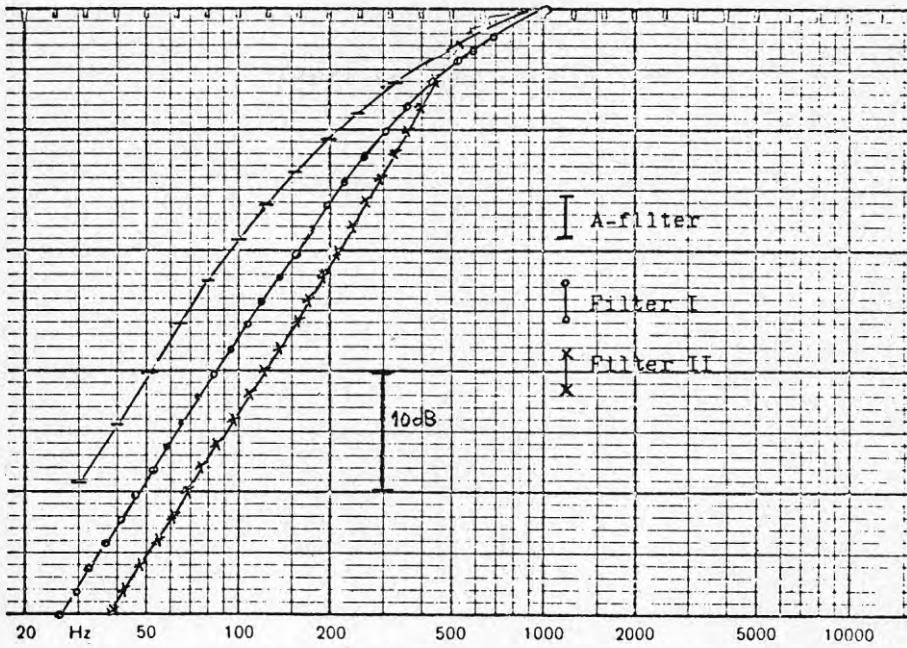
Figur Vågningsfilter för störnivå. Hörslingor.
