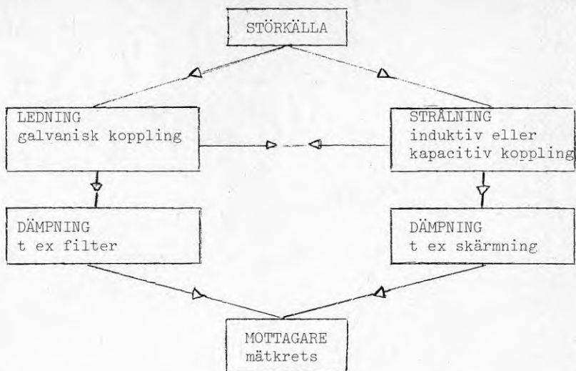
Fig. Störningars utbredning och dämpning
