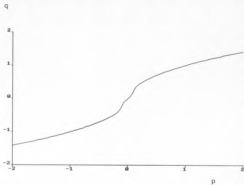
FIG.3.1 Två lika läckors nettoläckflöde q som funktion av referenstryckskillnaden p med z_1 = -z_2 = 0.1 .
