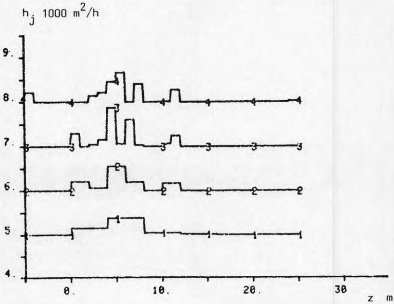
FIG. 6.8 Läckhöjder h_j , \text{m}^2/\text{h} för fyra rektangelformade läckprofiler som funktion av läget z m för en idrottshall.
