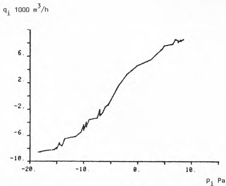
FIG. 6.2 Nettoläckutflöde q_i m 3 /h som funktion av inre övertryck p_i Pa för en idrottshall
