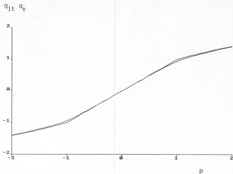
FIG.3.9 Läckflöde för en laminär-turbulent läcka q_{lt} och en rektangulär läcka q_r som funktion av referensstryckskillnaden p .
