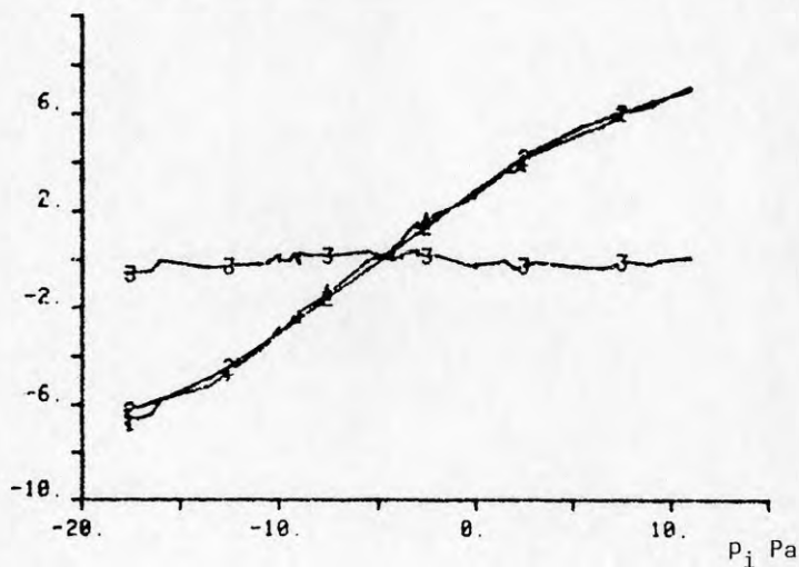
FIG.6.4 Verkligt och modellerat läckflöde q_i och q_{mi} och skillnad q_{ei} \text{m}^3/\text{h} som funktion av inre övertryck p_i Pa för modell S2.
