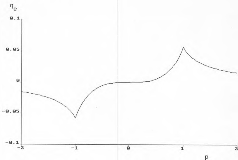
FIG.3.10 Skillnad i läckflöde mellan en laminär-turbulent och en rektangulär läcka q_e = q_{lt} - q_r som funktion av referensstryckskillnaden p
