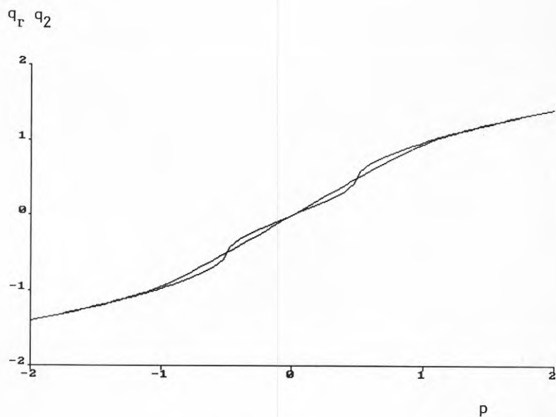
FIG.3.6 Läckflöde för en rektangulär läcka q_T och två punktformiga läckor q_2 som funktion av referenstryckskillnaden p
