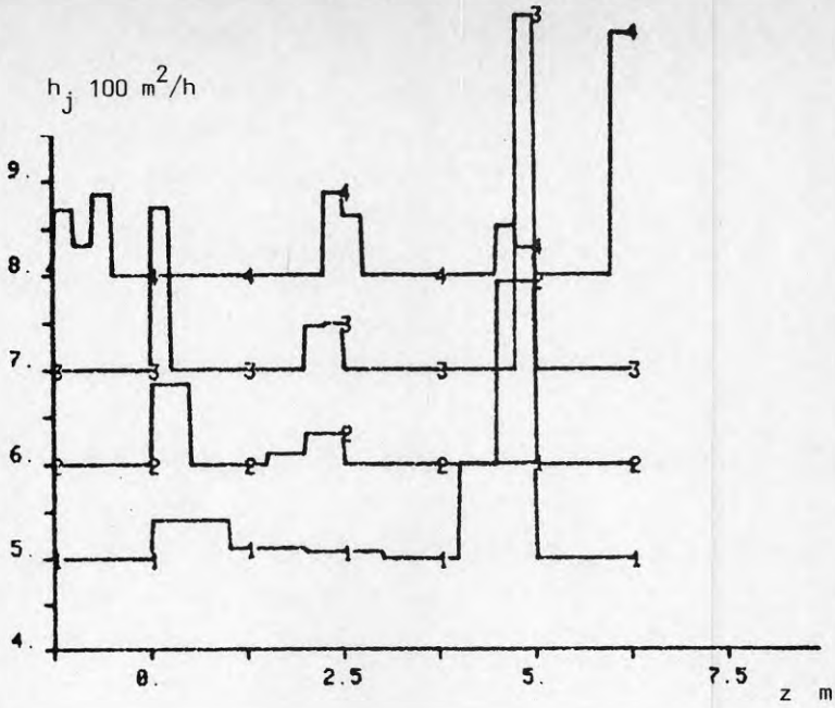
FIG. 6.7 Läckhöjder h_j , \text{m}^2/\text{h} för fyra rektangelformade läckprofiler som funktion av läget z m för ett småhus.
