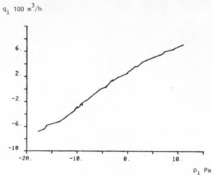
FIG. 6.1 Nettoläckutflöde q_i m 3 /h som funktion av inre övertryck p_i Pa för ett småhus
