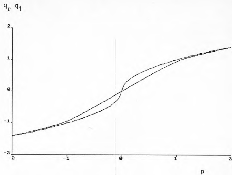
FIG.3.5 Läckflöde för en rektangulär läcka q_T och en punktformig läcka q_1 som funktion av referenstryckskillnaden p .
