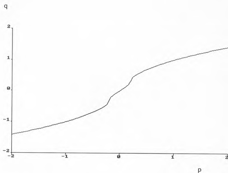
FIG.3.2 Två lika läckors nettoläckflöde q som funktion av referenstryckskillnaden p med z_1 = -z_2 = 0.2 .
