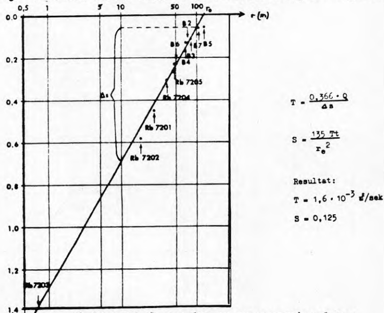
Figur 9.4. Avstånd-avsänkingsanalys av propvpumpningsdata.
