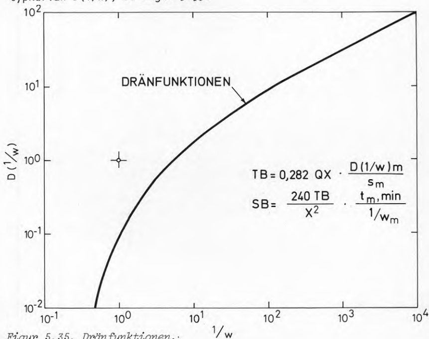
Figur 5.35. Dränfunktionen.
