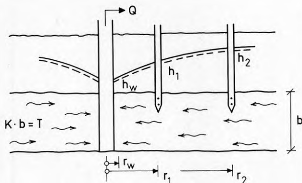
Figur 5.1. Radiellt flöde kring en brunn.
