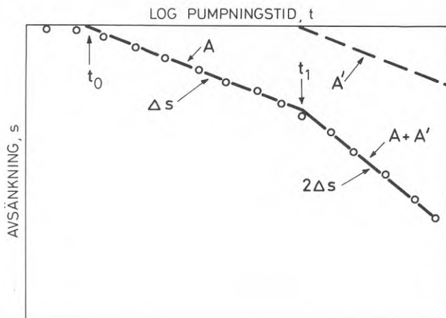
Figur 5.20. Avsänkingsförlopp vid negativ hydraulisk gräns.
