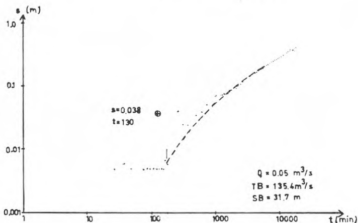
Figur 9.15. Datakurva för observationsrör 8.
