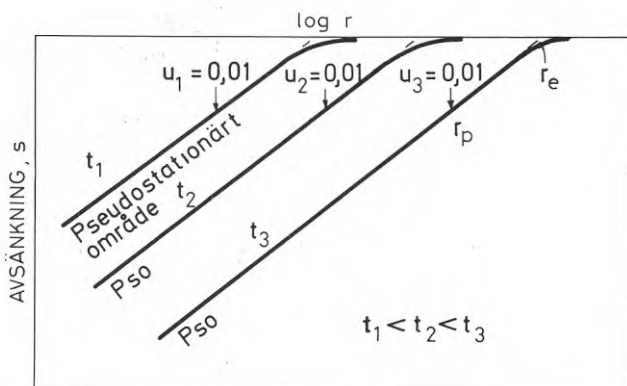
Figur 5.14. Avsänkningstrattens utbredning med tiden.
