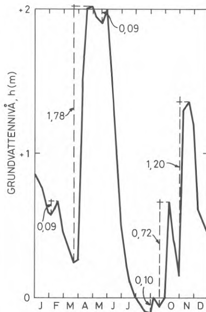
Figur 8.13. Grundvattennivåer 1969.
