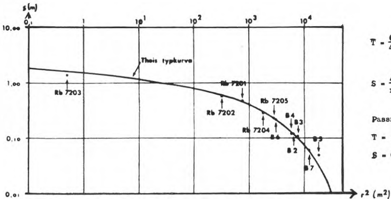
Figur 9.6. Avstånd-avsänkingsanalys av propumpningsdata.
