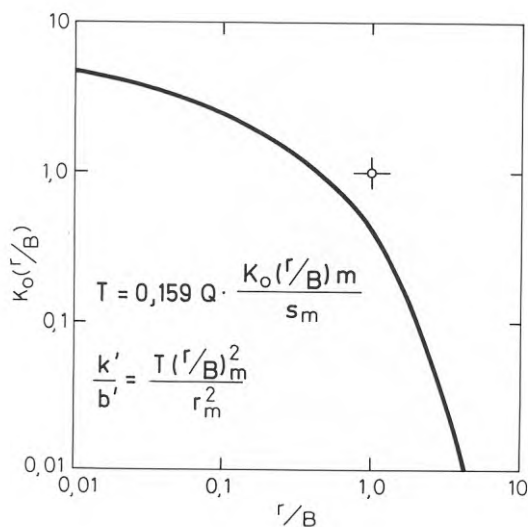
Figur 5.30. Typkurva K_0\left(\frac{r}{B}\right) .
