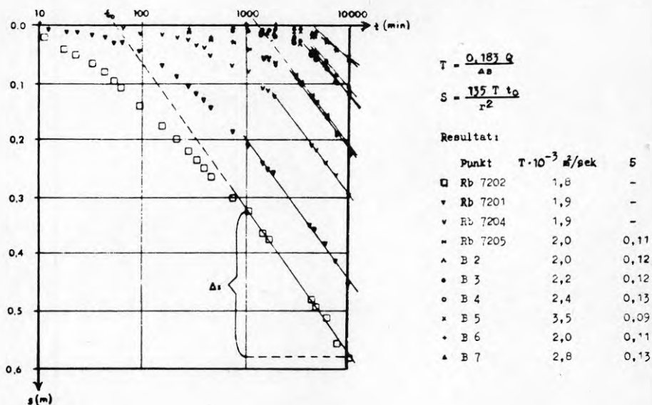
Figur 9.3. Tid-avsänkingsanalys av propvpumpningsdata.
