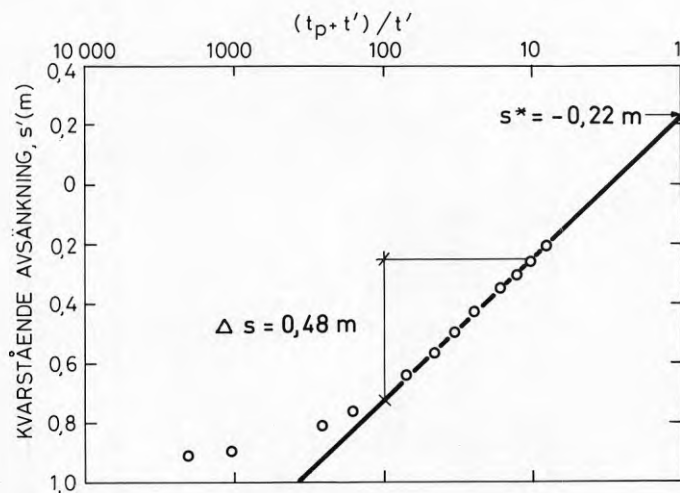
Figur 5.17. Analys av återhämtningsdata.
