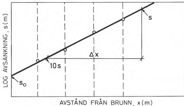
Figur 5.39. Avstånd-avsänkingsanalys för ås med läckage.
