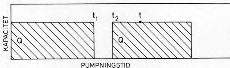
Figur 5.44. Uttag vid pumpning med pumpstopp.
