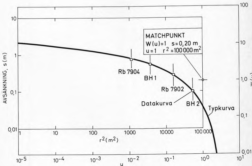
Figur 5.10. Avstånd-avsänkingsanalys genom kurvpasning.
