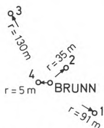
Figur 5.2. Obsrörens placering, se 5.1.
