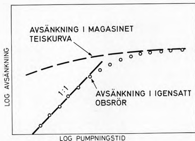
Figur 5.43. Avsänkingsförlopp i igensatt obsrör.
