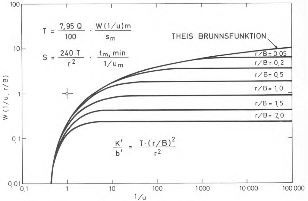
Figur 5.28. Theis-Waltons brunnfunktion W(1/u, r/B) .
