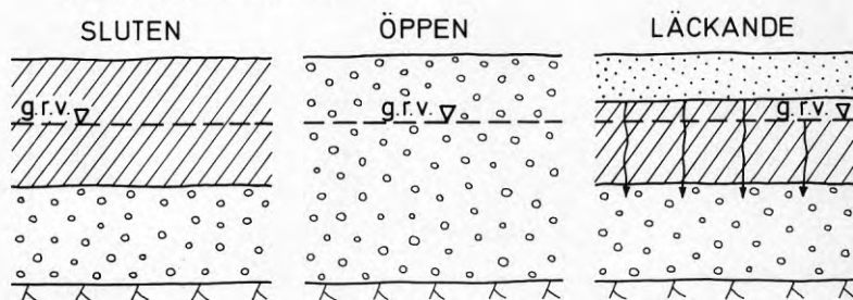
Figur 2.1. Principupbyggnad för sluten (a), öppen (b) resp läckande akvifer (c).
