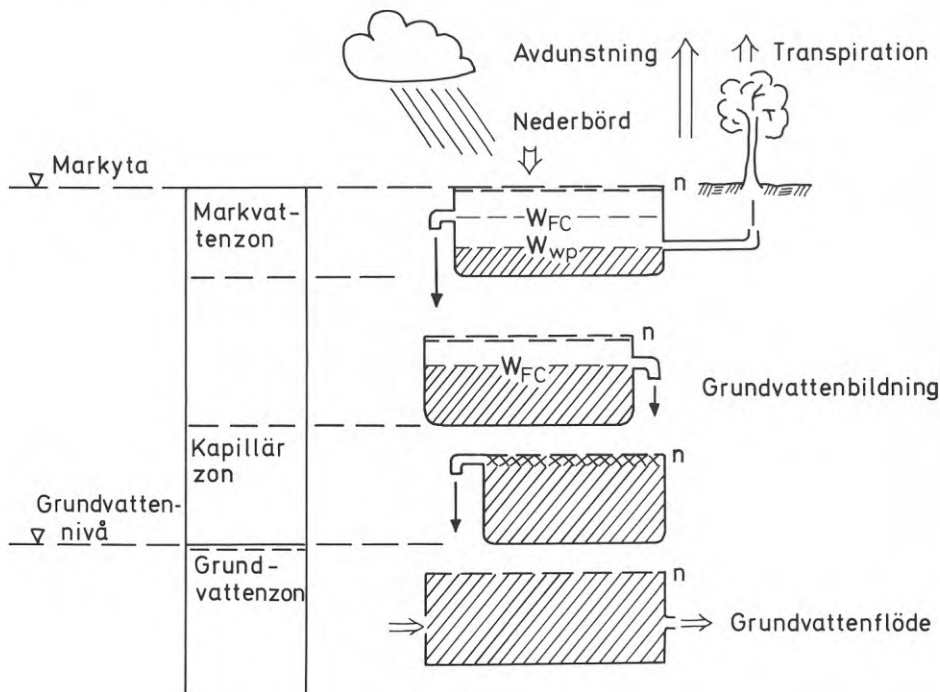
Figur 8.2. Underjordsvattnets magasinssystem.
