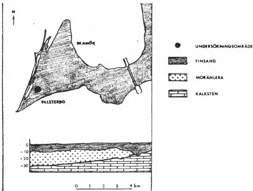
Figur 9.1. Geologisk karta över Falsterbohalvön, skala ca 1:130 000. I huvudsak efter hydrogeologiska kartblad Trelleborg NV och Malmö SV, Ser Ag Nr 4.
