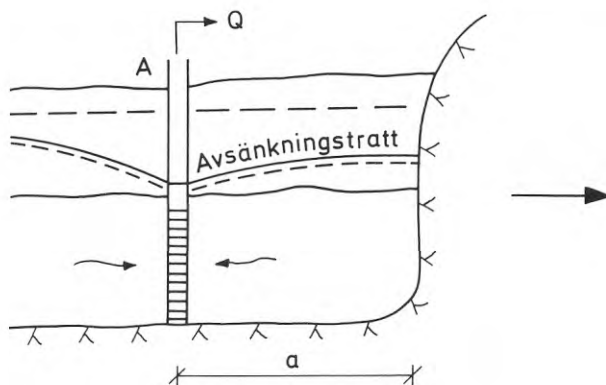
Figur 5.18. Pumpning intill negativ hydraulisk gräns.
