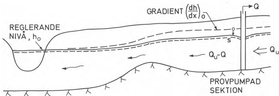
Figur 8.5. Avsänkning i en ås vid grundvattenuttag.
