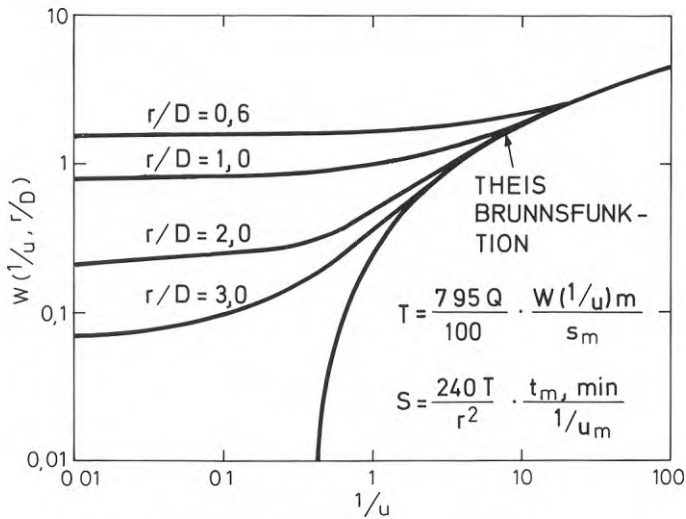
Figur 5.33. Theis-Boultons brunnsfunktioner.
