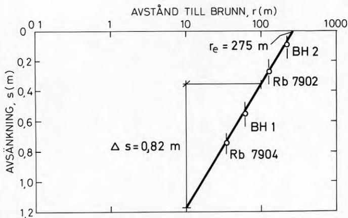
Figur 5.13. Avstånd-avsänkingsanalys, linlog.
