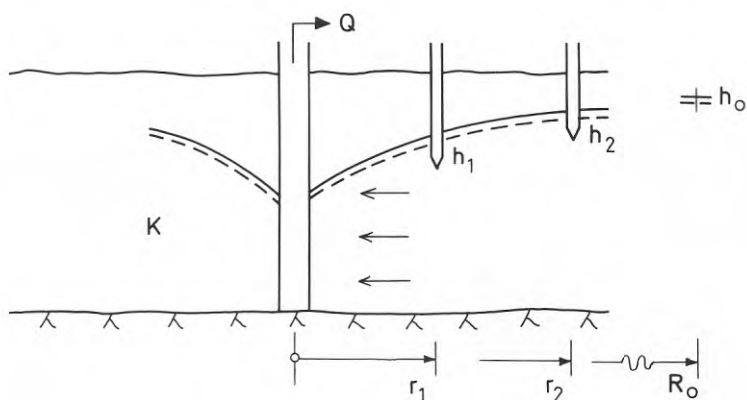
Figur 5.4. Flödet kring en brunn i ett öppet grundvattenmagasin.
