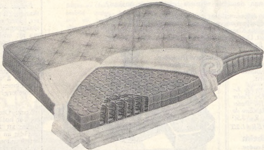
Dux-madrass med genomskärning. Under stoppningen framträder råstommen, i vilken man kan se de fristående Duxspiralerne inkapslade i celler. Flera hundra spiraler ingå i varje madrass.
