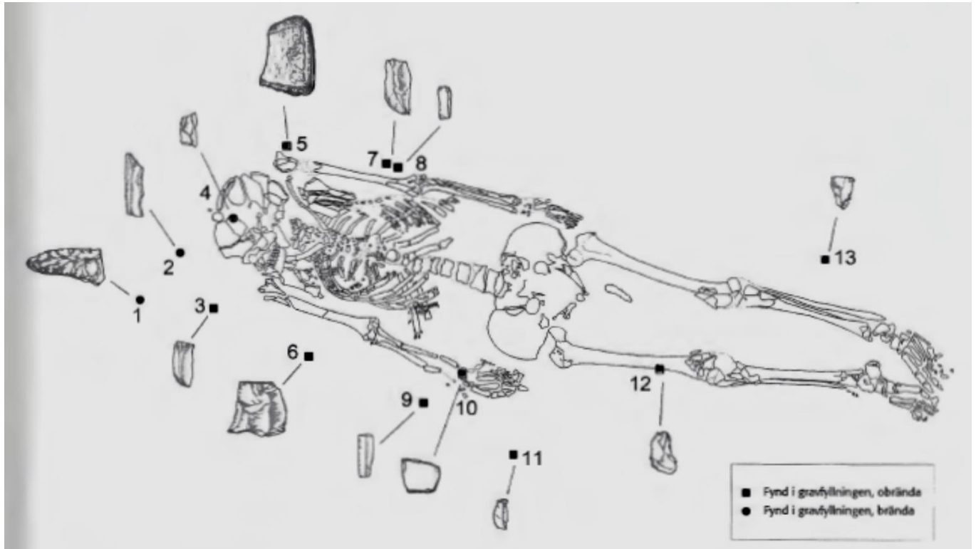
Figur 13 Artefakterna i grav 4 A6504: 1.Kärnyxa 2. Spån 3. Spån 4. Spån 5. Handtag 6. Polygonal kärna 7. Spån 8. Spån 9. Spån 10. Slipsten 11. Spån 12. Uppfriskningsavslag 13. Spån (Kjällquist 2001:47)
