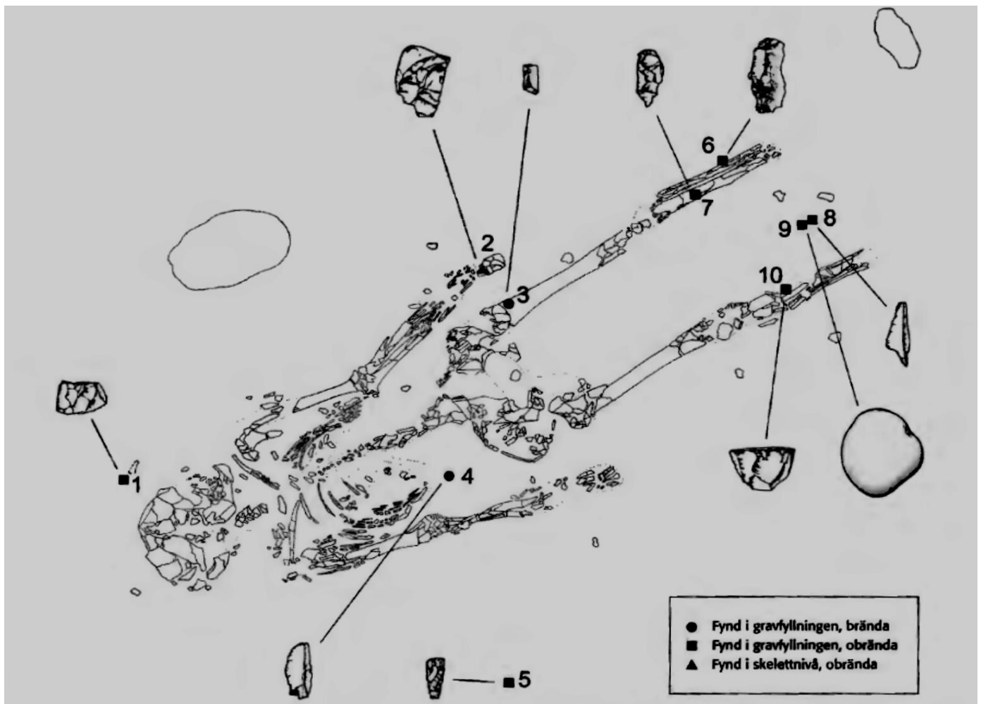
Figur 11 Artefakternas spridning Grav 1. 1. Handtagskärna 2. Polygonal kärna 3. Spån 4. Spån 5. Eldslagningsflinta 6. Spån 7. Uppfriskningsavslag 8. Spån 9. Knacksten 10. Handtagskärna (Kjällquist 2001:40)
