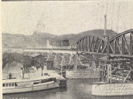
Öfverst: TRANSPORT AF BROSPANN Å PONTONER. Mellerst: VY AF BRON. Nederst t. v.: NORRA VIADUKTEN FRÅN LANDFÄSTET Å HISINGEN. Nederst t. h.: SÖDRA VIADUKTEN FRÅN LANDFÄSTET Å GÖTEBORGSSIDAN.
