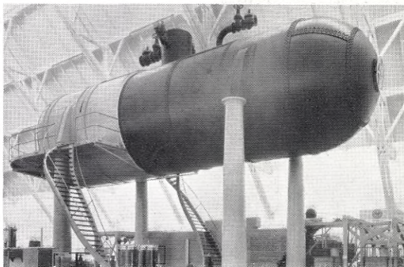
A.-B. VAPORACKUMULATOR. DR. RUTHS' ACKUMULATOR Å JUBILEUMSUTSTÄLLNINGEN I GÖTEBORG.
