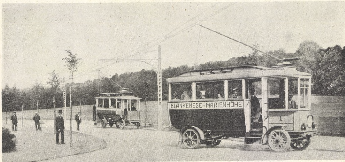
OMNIBUSTRAFIK MED ELEKTRISK LUFTLEDNING, nyligen insatt på en vägsträcka i Tyskland — en projekterad möjlighet i Helsingborg.
