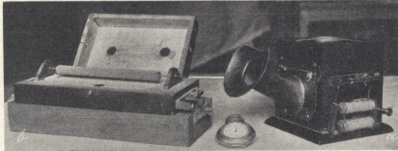
Efter fotografi. Kliche: Bengt Sjöqvistsparre. REIS 1863 FÖRBÄTTRADE TELEFONAPPARAT: a afsändaren, b mottagaren.
