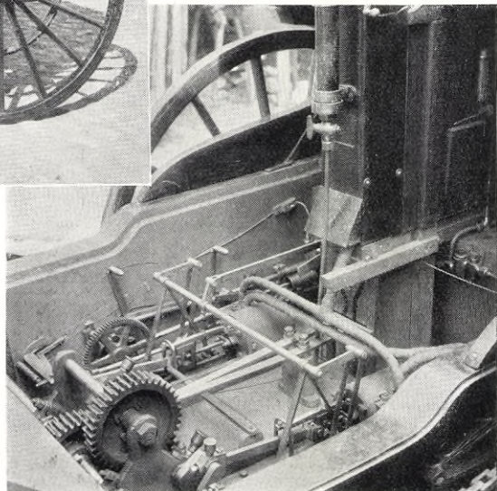
MOTORMEKANISMEN.
