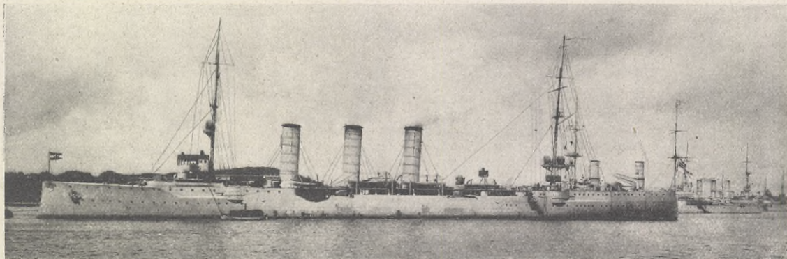
KAMPEN OM HERRAVÄLDET ÖFVER HAFVET: Den nybyggda tyska kryssaren "Kolberg", längd 120 m., bredd 14 m., djugaende 5 m.; om 4,300 tons; 16 kanoner, 300 mans besättning.
