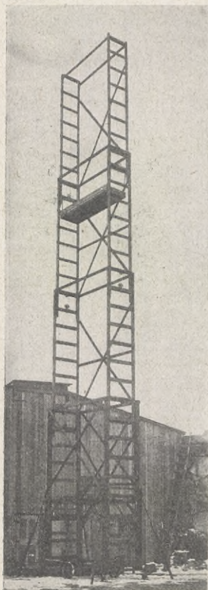
H. 8 Da STOCKHOLMSFOTOGRAF. INGENIÖR J. W. CARLSSONS HÖJ- OCH SÄNKBARA BYGG- NADSSTÄLLNING.
