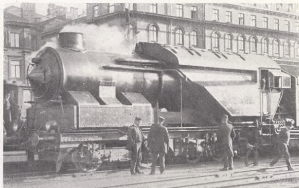
Vidstående bild: DET FÖRSTA SVENSKA TURBINLOKOMOTIVET Å STATSBANORNA. Foto Norborg, Sthlm.
