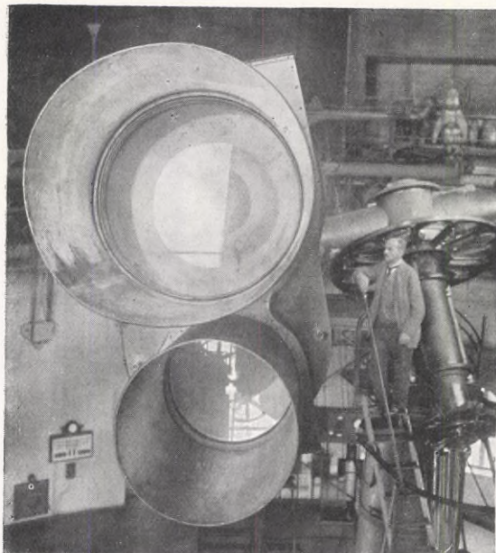
Efter fotografi. POTSDAM: OBJEKTIVÄNDAN AV KIKAREN med de båda gigantiska linserna — den övre till den fotografiska plåten. Kikare: Sjoberg, Gbg.
