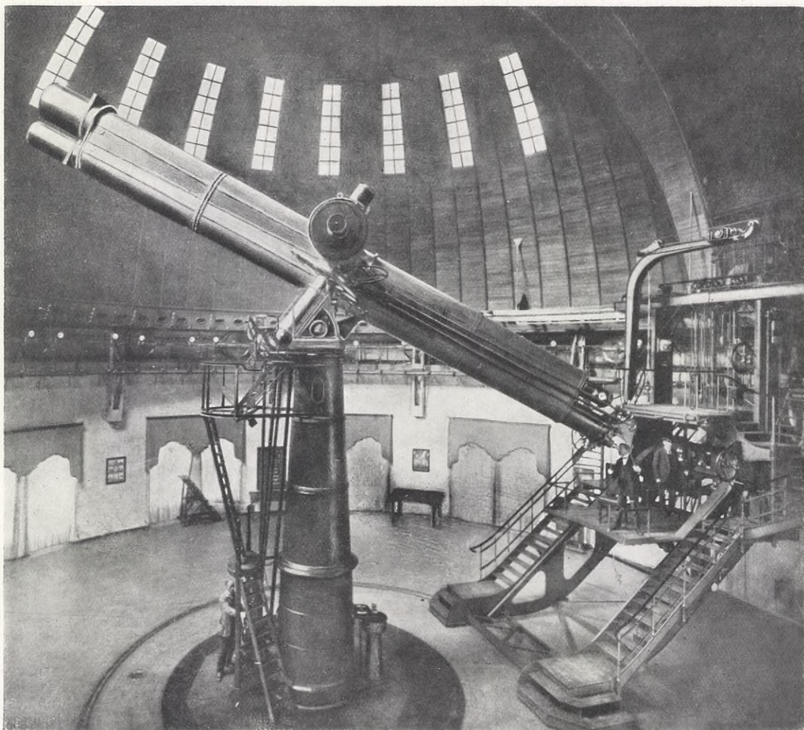
DEN STORA DUBBELREFRAKTORN, 12 m. lång med rörlig observationsbalkong (t. h.). Bakom observatören vid kikarens okularända synes en medhjälpare vid den elektriska kopplingstavlan, från vilken de erforderliga rörelserna hos observationsbalkongen, taket och kikaren dirigeras. — Efter fotografier. — Kliché: Sjöberg, Gbg.
