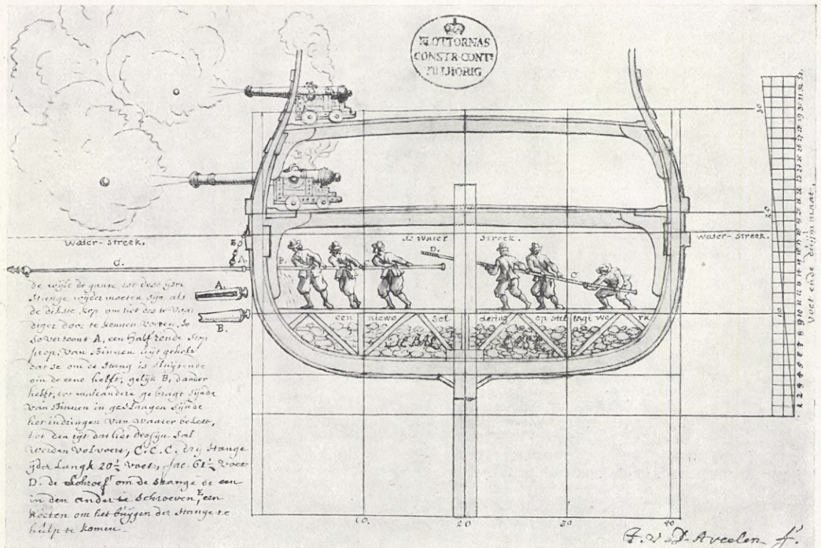
ETT ÖRLOGSFARTYGG MED ETT SPJUTLIKNANDE FÖREMÅL GENOM FARTYGGSIDAN UNDER VATTENLINJEN — möj- ligen en föregångare till den omkring 200 år senare uppfunna stångtorpeden. Efter en samtida teckning i ett svenskt sjömilitärt arkiv. — Kliché: Aug. Sjöbergs Klichéanst., Gbg.
