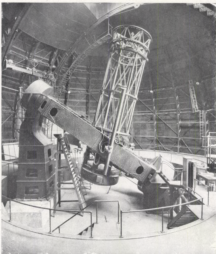
FIG. I. VÄRLDENS STÖRSTA TELESKOP Å MOUNT WILSONOBSERVATORIET I CALIFORNIEN, varmed de följande månfotografierna äro tagna. Teleskopets brännspiegel har en diameter av 2\frac{1}{2} meter.
