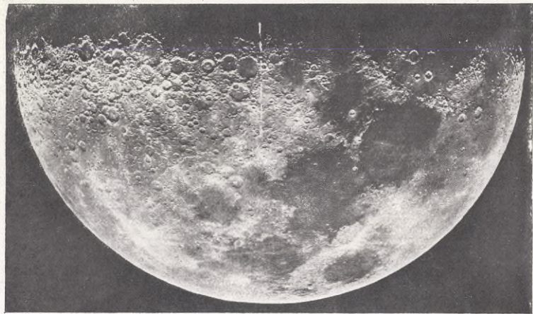
FIG. V. FOTOGRAFI AV MÅNEN I "FÖRSTA KVARTERET", tagen med Potsdamobservatoriets stora fotografiska tub, Europas största. Mount Wilsonteleskopets atomordentliga överlägsenhet torde framgå av jämförelsen mellan denna bild och de i fig. II—IV återgifna. Samtliga månbilder äro förmånskaade i samma pro-
