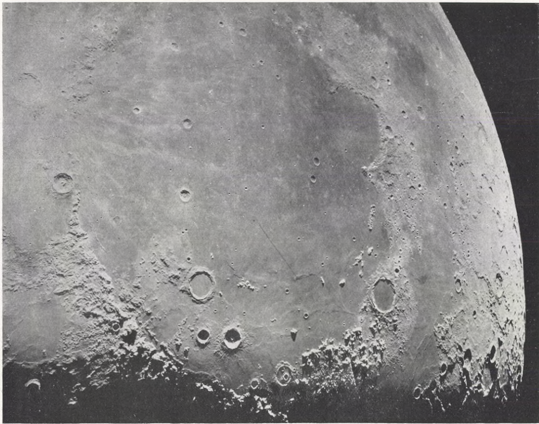
FIG. III. FOTOGRAFI AV "MÅNHAVET" MARE IMBRIUM — det stora slåta området — med omgivning. Längst upp: ringberget Kopernikus och t. v. Mån-Apeninernas väldiga bergskedja; nederst: norra månranden. Den s. h. "regnbågshukten", ligger 2 1/2 cm. nedom mitten t. h. Landskapet framträdet kanske bäst om man vänder upp och ned på bilden. — Bild: Gode Zilberd & Krichmannski, Öpp.
