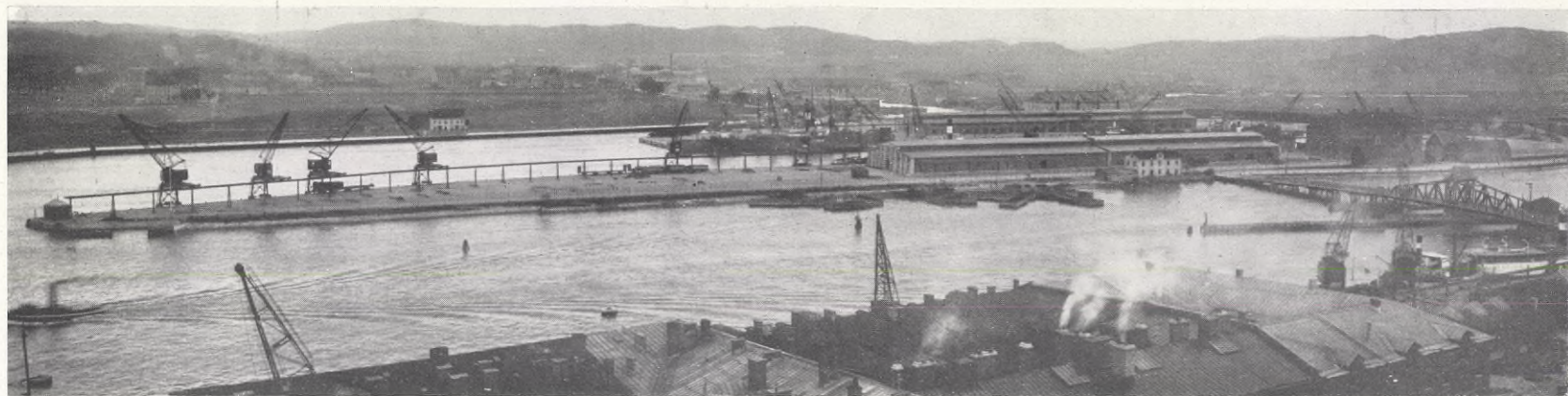
GÖTEBORGS NYA FRIHAMN, CENTRALHAMNEN, inviges den 31 augusti. Hela den stora hamnantagningen kommer att draga i kostnader 21,475,000 kronor; det inhägnade området är 38,4 hektar, varav 18,6 land. Genom Hisingsbron står frihamnen i landförbindelse med staden. — Text å sid. 781. — Foto. Allard, Gbg — Klisché: Göes Bildbyrå & Klischéanstalt, Gbg
