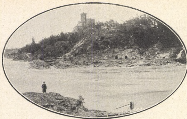
LÄGET VID »OLIDEHÅLAN» FÖR DEN BLIFVANDE KRAFTSTATIONEN. I bergväggen synas utsprängda tuber för vattnets ledande från kraftkanalen ned till turbinerna i kraftstationen.
