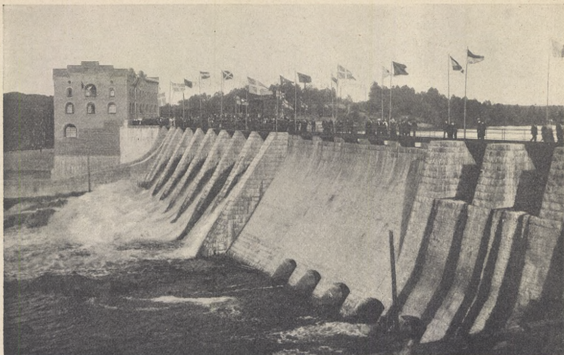
Foto. Widén Laholm. ÖFRE KNÄREDS KRAFTSTATION I FESTSKRUD INVIGNINGSDAGEN.
