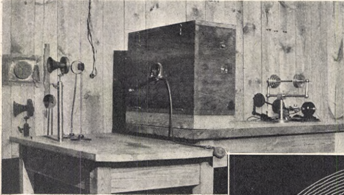
FOTOGRAFONENS MOTTAGNINGSPPARAT.
