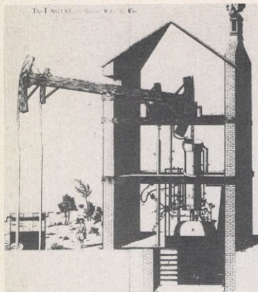
Newcomens ångmaskin. Kopparstick från år 1725.
