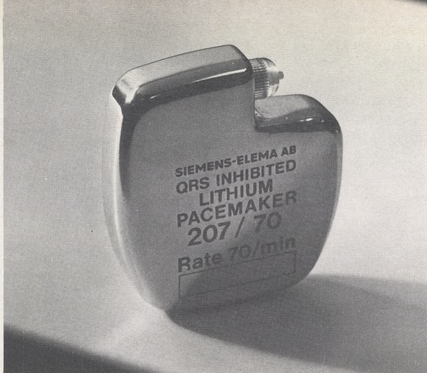
Så här ser en modern pacemaker ut. Den drivs av ett litium-jodid-batteri.
