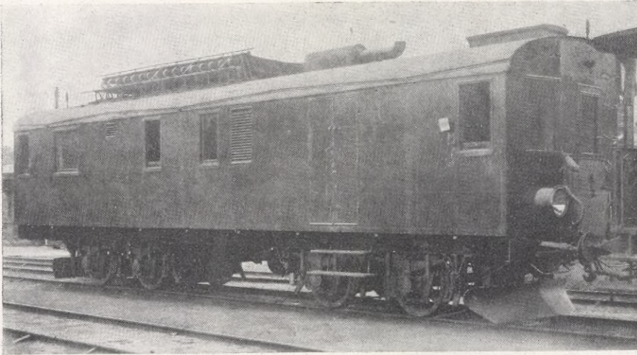
DIESEL-ELEKTRISK MOTORVAGN LEVERERAD AV ALLM. SVENSKA ELEKTRISKA A.-B., VÄSTERÅS till Dieselektriska Vagnaktiebolaget . — Efter fotograf.
