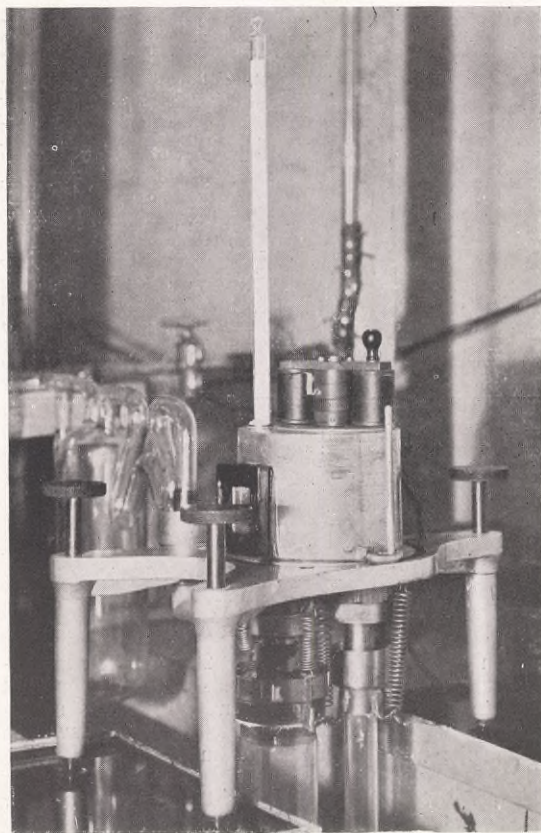
T. v. MIKROVÅGEN UTAN OCH (överst t. h.) MED SKYDDSLÖCK. Nederst: SCHEMATISK FRAMSTÄLLNING AV MIKROVÅGEN. — Kliché: Coës, Gbg.
