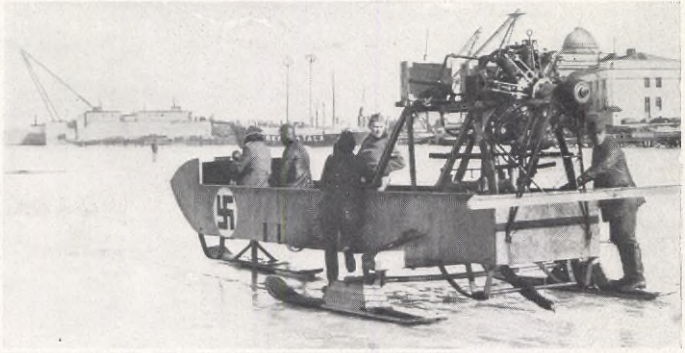
EN ORIGINELL MOTORSLÄDE försedd med aeroplanmotor och propeller, avsedd för 10 personer vid färden från och till Sveaborg.
