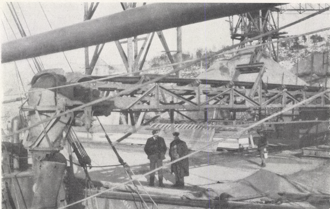
SULITELMA: Svafvelkisen in'astas i Fineidet, Sulitelmas uthamn, medelst högmoderna anordningar, som kunna lasta 1200 ton på omkr. 18 timmar. — Amatörfoto P. Carlberg, Stockholm.
