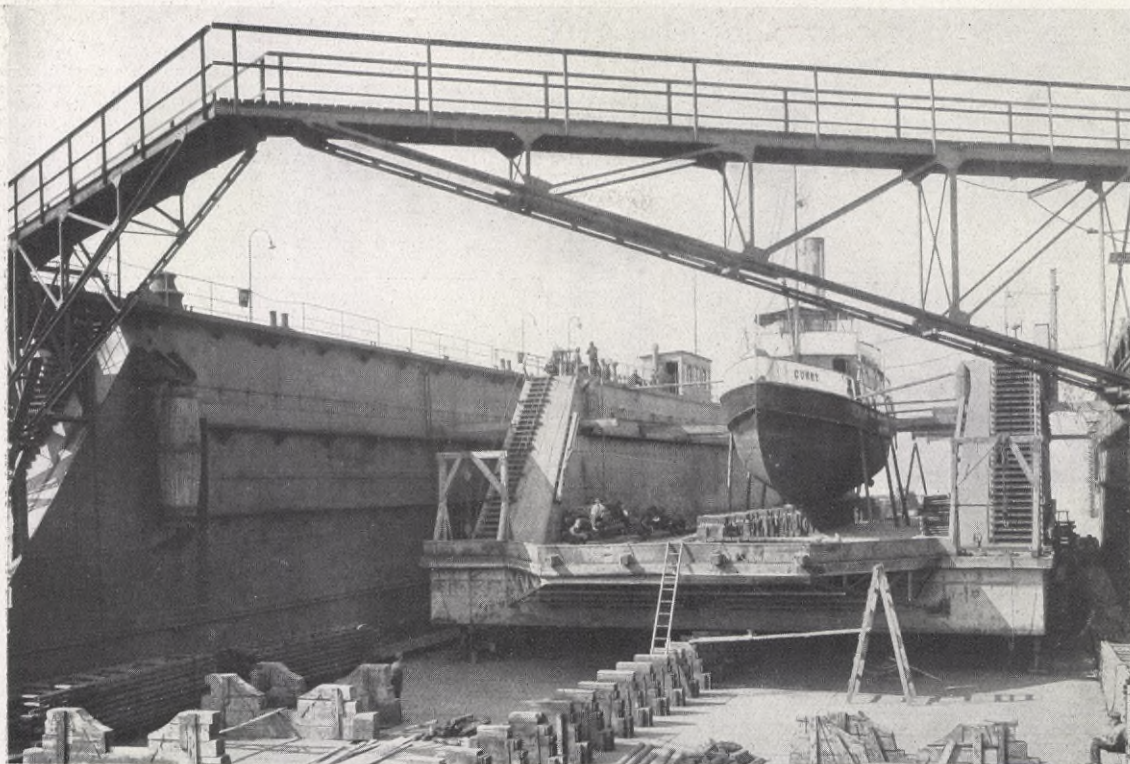
GÖTAVERKENS JÄTTEDOCKA UNDERGÅR ETT ENASTÅENDE PROF: upptager i sig Eriksbergs flytdocka med däri till reparation intagen ångare. Text å sid. 587.
