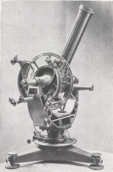
Efter fotografi 6. VERTIKALCIRKEL, ett instrument, hvärmed man noggrant fixerar himlakropparnes läge på himlen.
