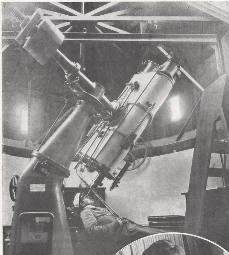
3. ASTROGRAFEN, anskaffad 1914 till större delen med tillhjälp af medel som donerats till Observatoriet af en gifvare, som önskat vara okänd. Detta instrument är uppställt i ett särskildt torn i observatorieträdgården.
