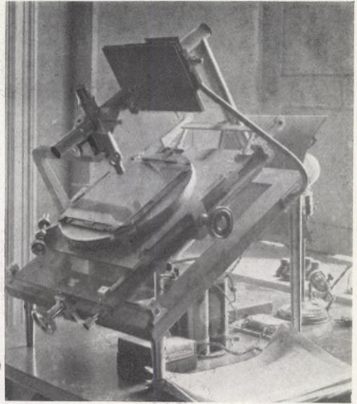
Efter fotografi 7. FRÅN RÄKNEKAMMAREN. Mikrofotometer enligt Haartmanns princip, nu använd vid de stellarstatistiska arbeten öfver stjärnfördelningen i Vintergatan, som för närvarande pågå vid Observatoriet.
