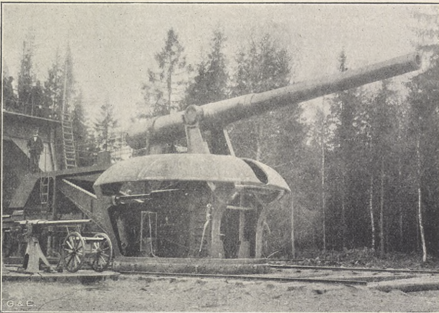
BOFORS: Den stora 24-cm -kanonen, färdig till skjutning. Den största i Sverige tillverkade kanon; afsedd för Oscar-Fredriksborgs fästning.
