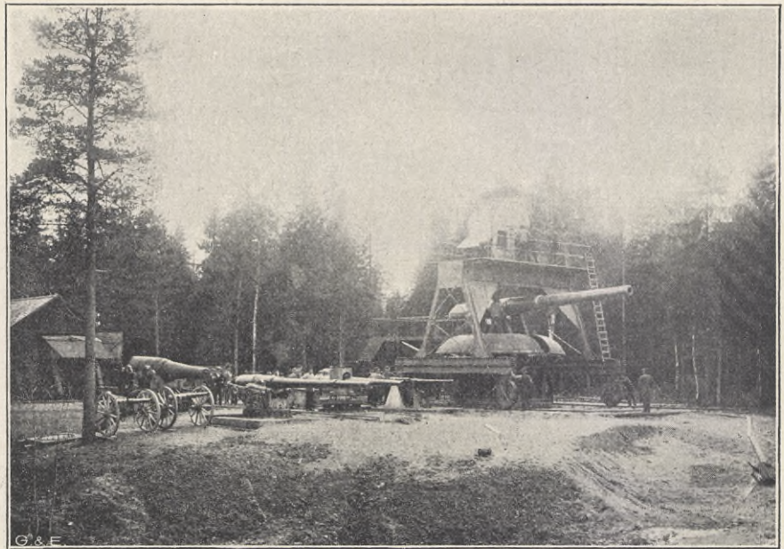
BOFORS: Skjutplatsen, med den stora 24-cm-kanonen till höger.
