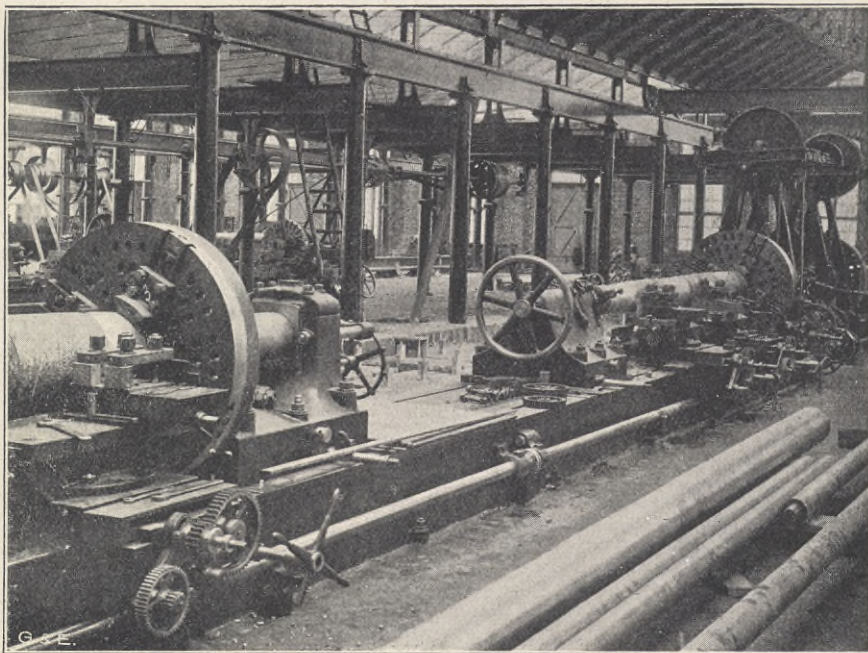
BOFORS: Interiör af kanonverkstaden. Man ser kanonännena i svarfvarne.
