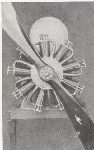
ROTATIONSMOTOR PÅ 80—100 HK. af Thulins konstruktion och tillverkning — modifikation af fransk motor.
