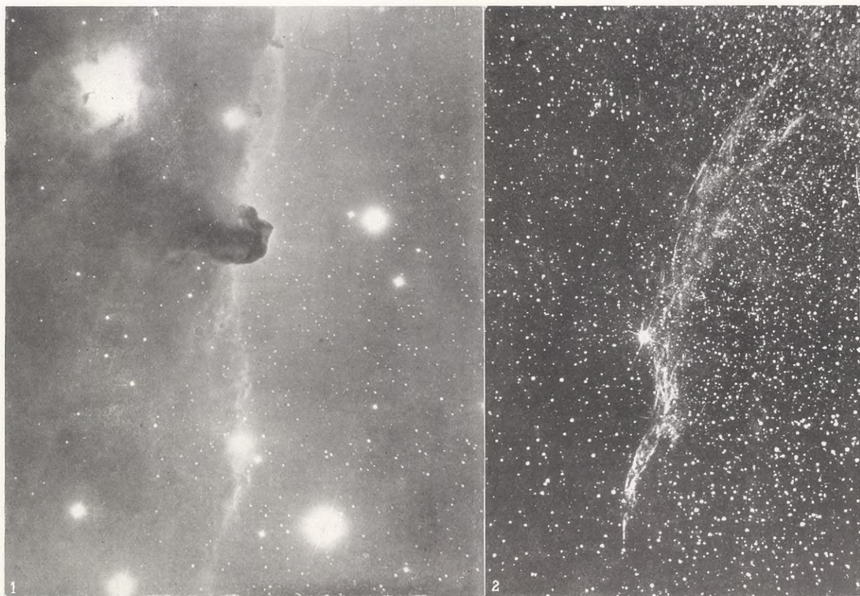
Fig. 2. Mörk nebulosa, lysande i högra randen, belägen invid stjärnan 52 i Svanen (mitt å bilden). Det mörka molnet framträder genom stjärnfattigdomen t. v. Efter originalfotografi, erhållen från prof. Max Wolf i Heidelberg.
