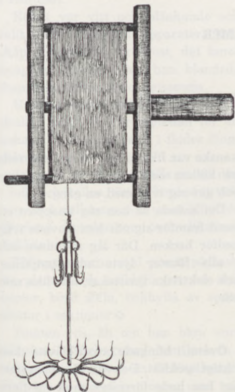
Granvinda med krokar för lukbusfiske. Betet sitter på de övre krokarna, krokkrönan hugger laken i buken, fångar den
