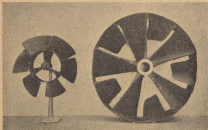
"Flygfiskens" propeller enligt John Ericssons typ samt t. h. ångfartyget "Jönköpings" propeller enligt O. E. Carlsunds konstruktion från år 1846. Propellrarna äro uppställda i Tekniska Museets maskinhall i Stockholm.
